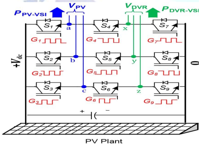
Fig.4: Sag Mode
